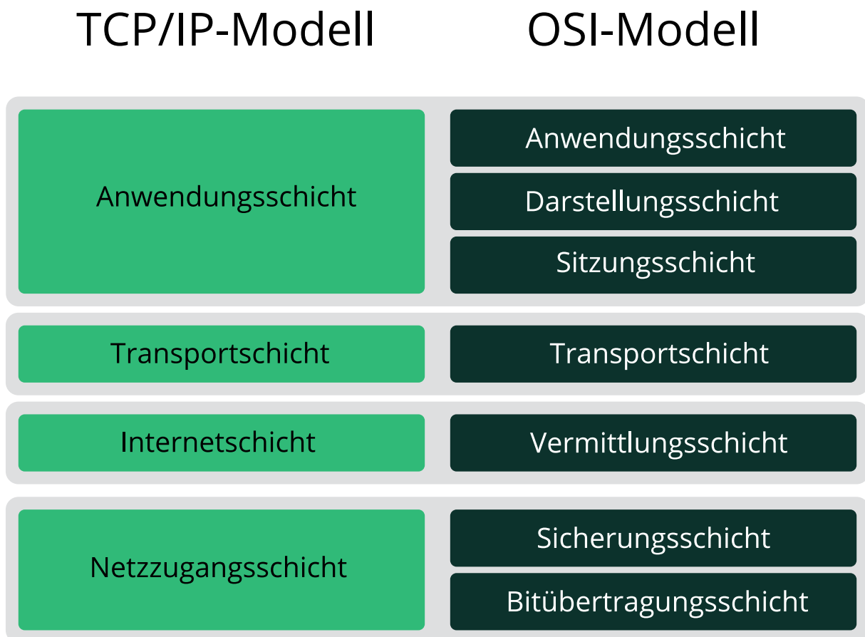
ABBILDUNG 23.1: VEREINFACHTES SCHICHTMODELL FÜR TCP/IP
