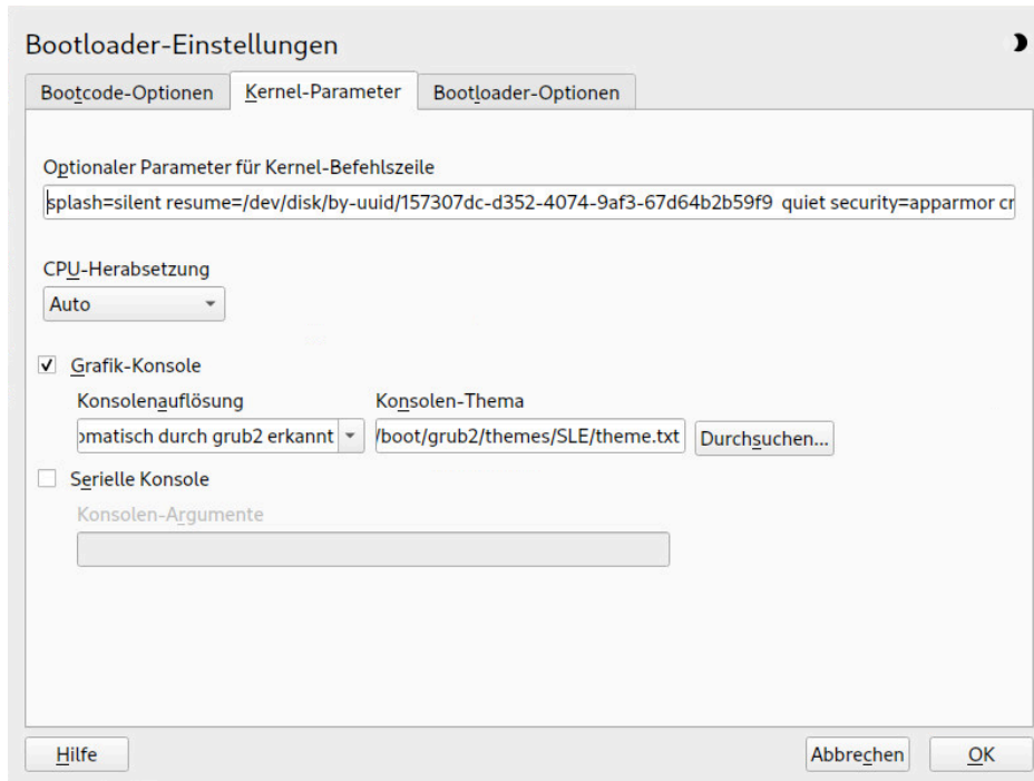
ABBILDUNG 18.4: KERNEL-PARAMETER
