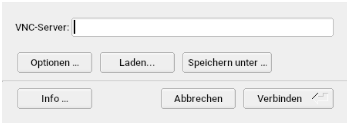
ABBILDUNG 14.1: VNCVIEWER
