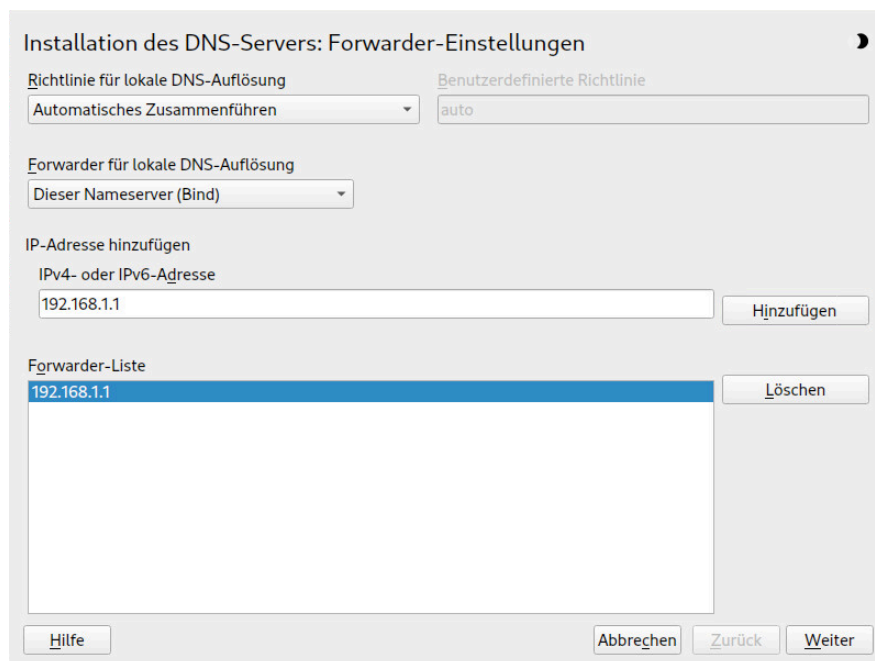
ABBILDUNG 39.1: DNS-SERVER-INSTALLATION: FORWARDER-EINSTELLUNGEN
