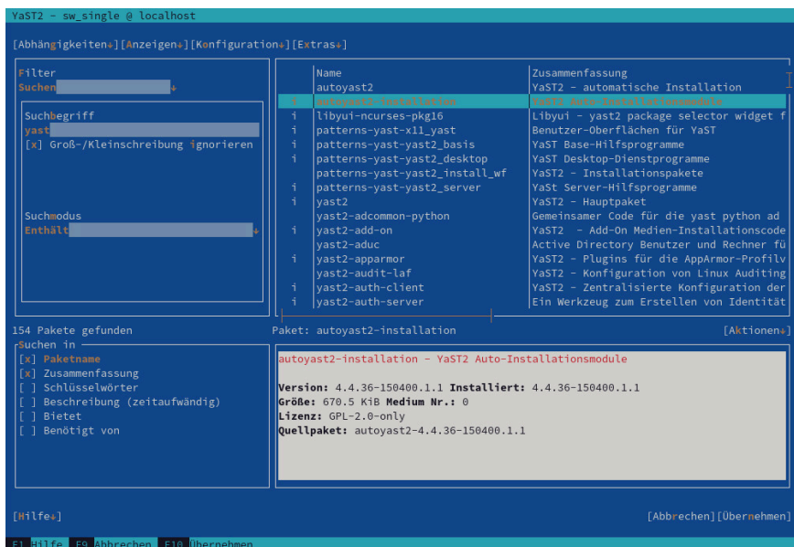
ABBILDUNG 4.2: DAS SOFTWARE-INSTALLATIONSMODUL
