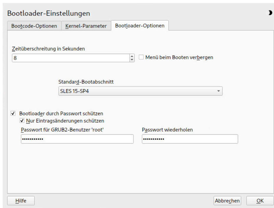
ABBILDUNG 18.3: BOOTLOADER-OPTIONEN
