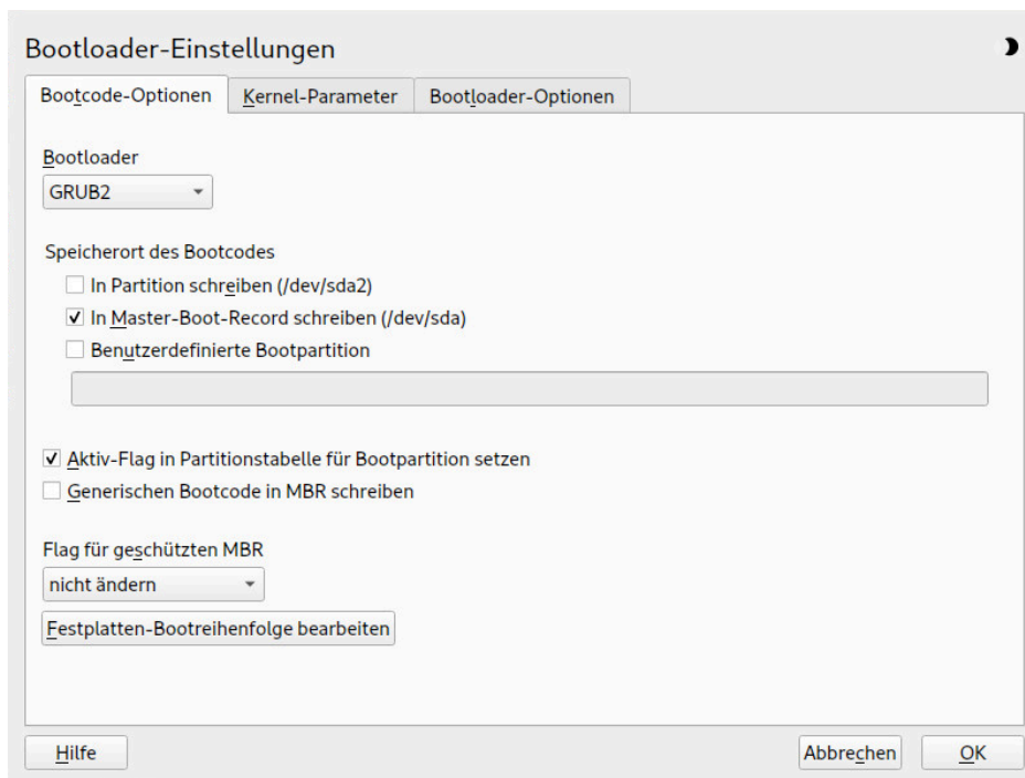
ABBILDUNG 18.2: BOOTCODE-OPTIONEN
